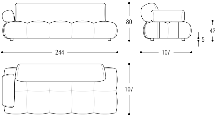
Element cm 244 left
