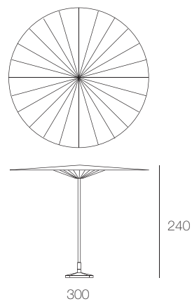
CA09C flat parasol
